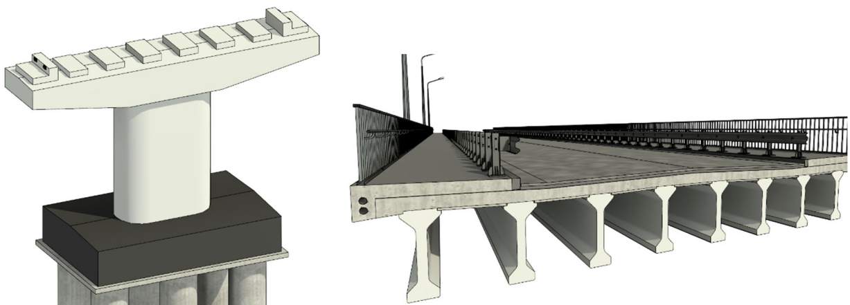
Рисунок 6 – Візуальне представлення цифрових моделей елементів мосту.
