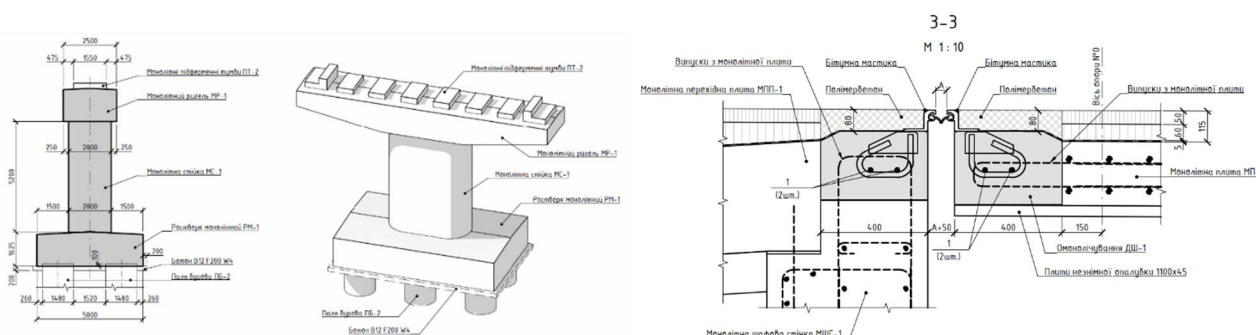
Рисунок 8 – Елементи та вузли конструкції мосту оформлені в Autodesk Revit. Figure 8 – Bridge structure elements and details drawn up in Autodesk Revit.
