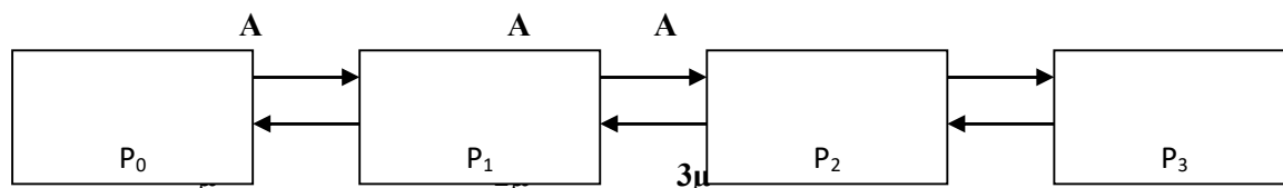
Рисунок 2 – Граф станів СМО з відмовами
