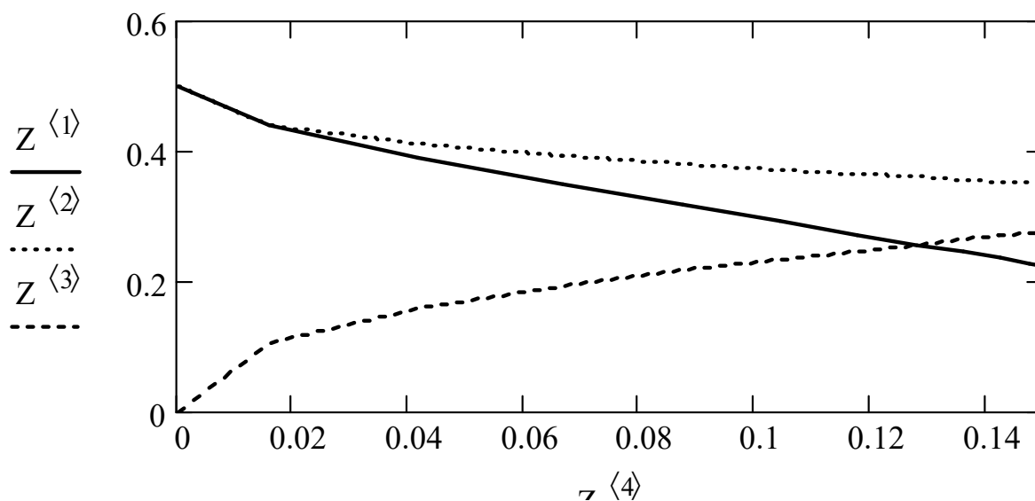
Рисунок 4 – Відносна динаміка зміни станів СМО Figure 4 - Relative dynamics of GS state changes
