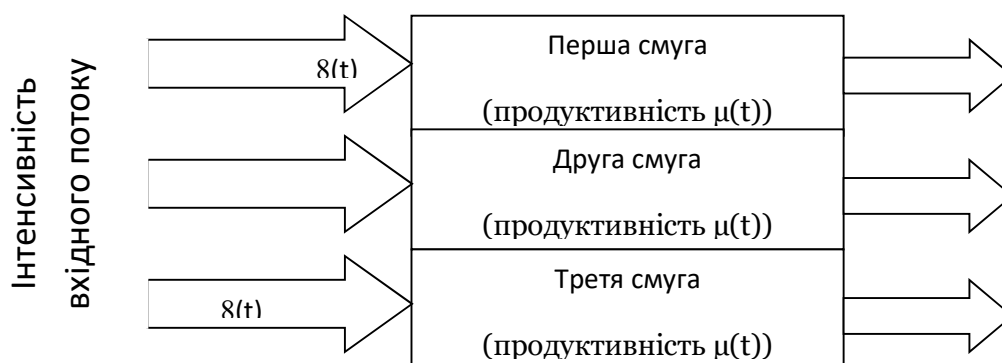
Рисунок 1 – Структурна схема ділянки дороги, представленої як СМО
