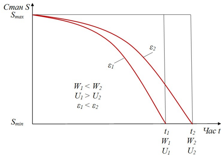
Рисунок 1 – Гіпотетичний вплив різних зусиль підрядника на стан елементу дороги Figure 1 - Hypothetical influence of different contractor efforts on the road element condition
