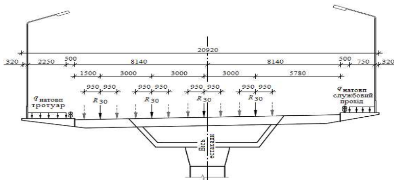
Рисунок 3 – Схема прикладення складових тимчасового навантаження до поперечного перерізу прогонової будови естакади спряження
