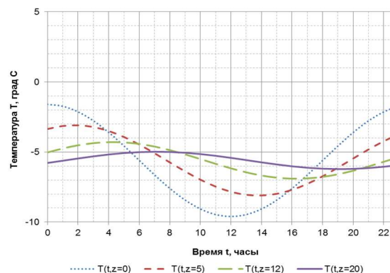
Рисунок 3 – Зміна температури в шарах дорожнього одягу в зимовий період
