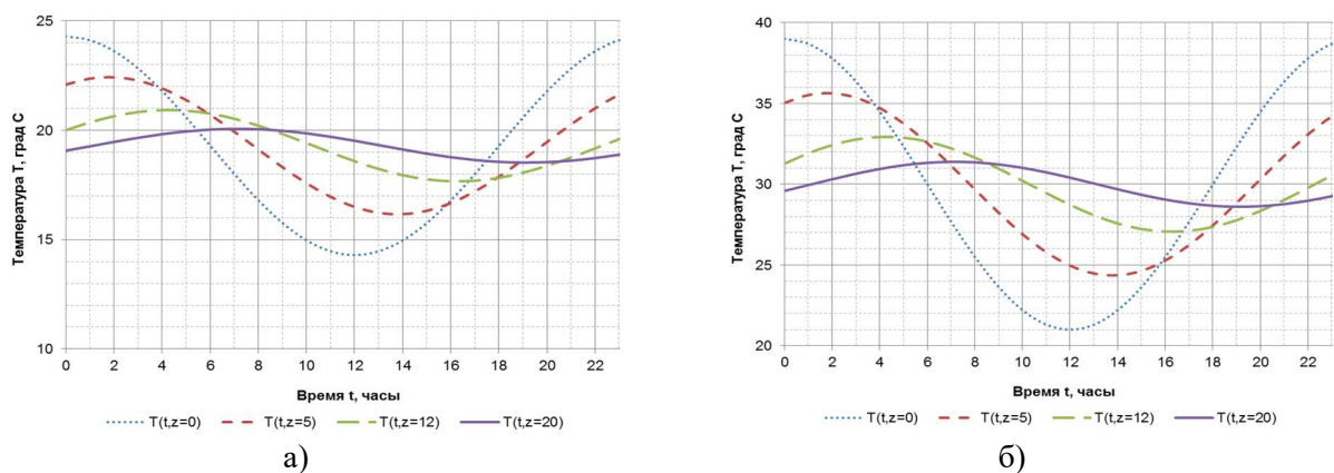
Рисунок 1 – Зміна температури в шарах дорожнього одягу в літній період: а) - при нормальних температурах; б) - при підвищених температурах
