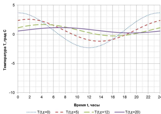
Рисунок 4 – Зміна температури в шарах дорожнього одягу у весняний період
